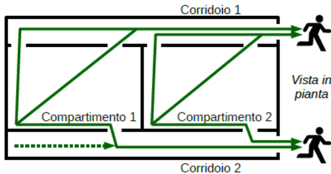
Illustrazione S.4-4: Esempi di vie d'esodo orizzontali ed uscite indipendenti
